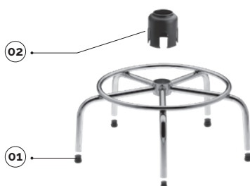
b30-base per sgabello con anello poggipiedi cono Ø50 tappi esclusi b30-base for stool with footrest ring cone Ø50 caps excluded
