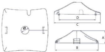
08 cpg-copertina in plastica per telaio girevole cpg-plastic cover for swivel frame
