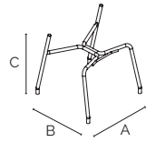
18 genesis - telaio 4 gambe con fori per cestello porta oggetti per ruote e piedini alti genesis - fixed 4 legs frame with holes for storage basket for castors and long glides
