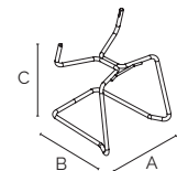
23 genesis - base a slitta in tubo asform d.22 tappi esclusi genesis - cantilever frame asform pipe d.22 without caps
