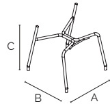
17 genesis - telaio 4 gambe per ruote e piedini alti genesis - fixed 4 legs frame for castors and long glides
