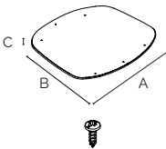
15 forma - pannello sedile in multistrato di betulla tappezzabile per scocca in plastica - viti di fissaggio incluse forma - upholsterable birch plywood seat panel for plastic shell - fixing screws included
