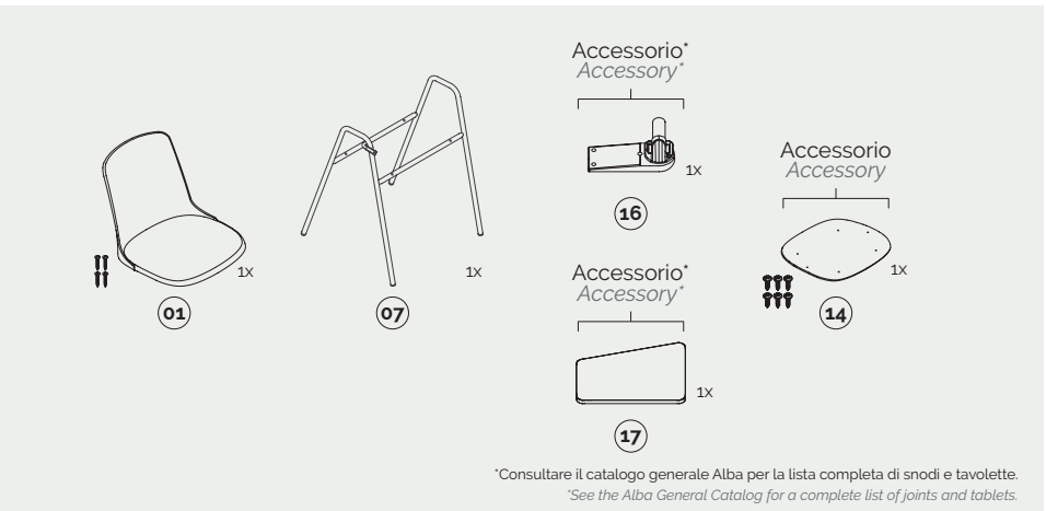
kit 4 gambe con braccioli e porta-tavoletta / 4-leg with armrests and tablet-holder
