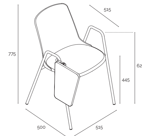
versione 4 gambe con braccioli e porta-tavoletta 4-leg version with armrests and tablet-holder
