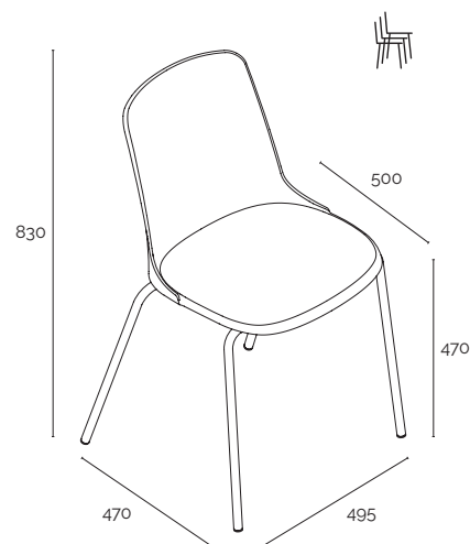
versione 4 gambe 4-leg version
